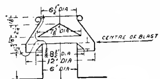
Fig. 4310. THE STASCH.
